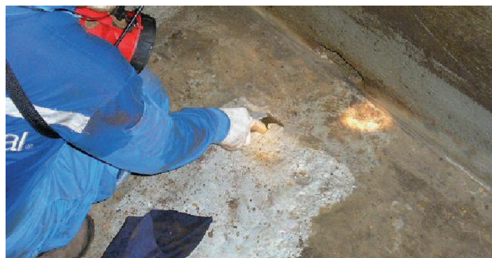
Днище резервуара для сырой нефти с питтинговой коррозией – 6 лет эксплуатации. Общее состояние Intershield 300 прекрасное несмотря на грязь и нефтяные пятна.
